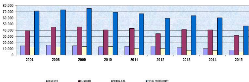
EVOLUCION DEL TRAFICO DE PRODUCTOS DE LA CONSTRUCCION EN MILES DE TON-KMS
